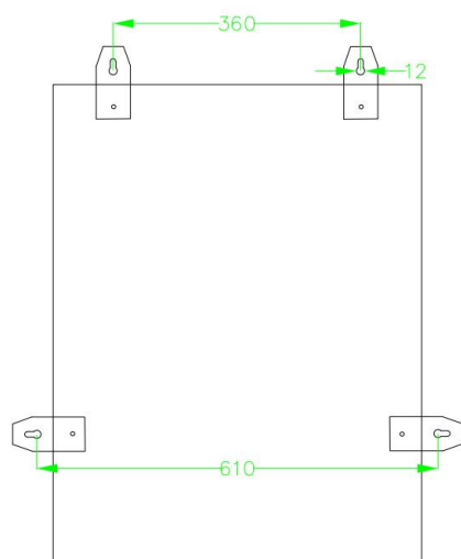
背面安装孔
