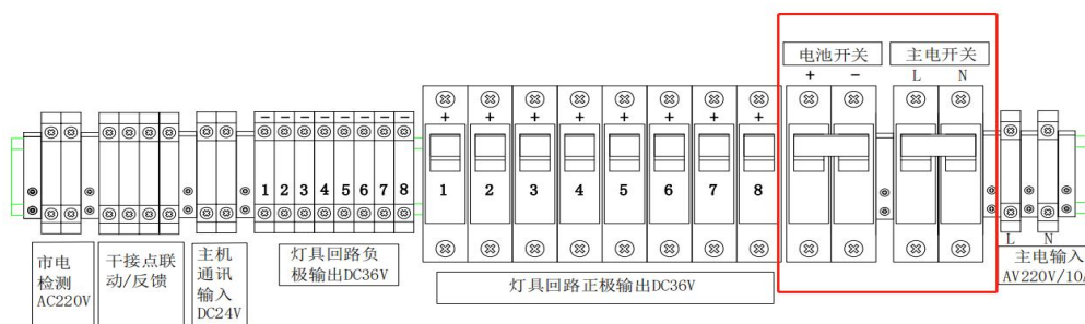
1:回路开关
